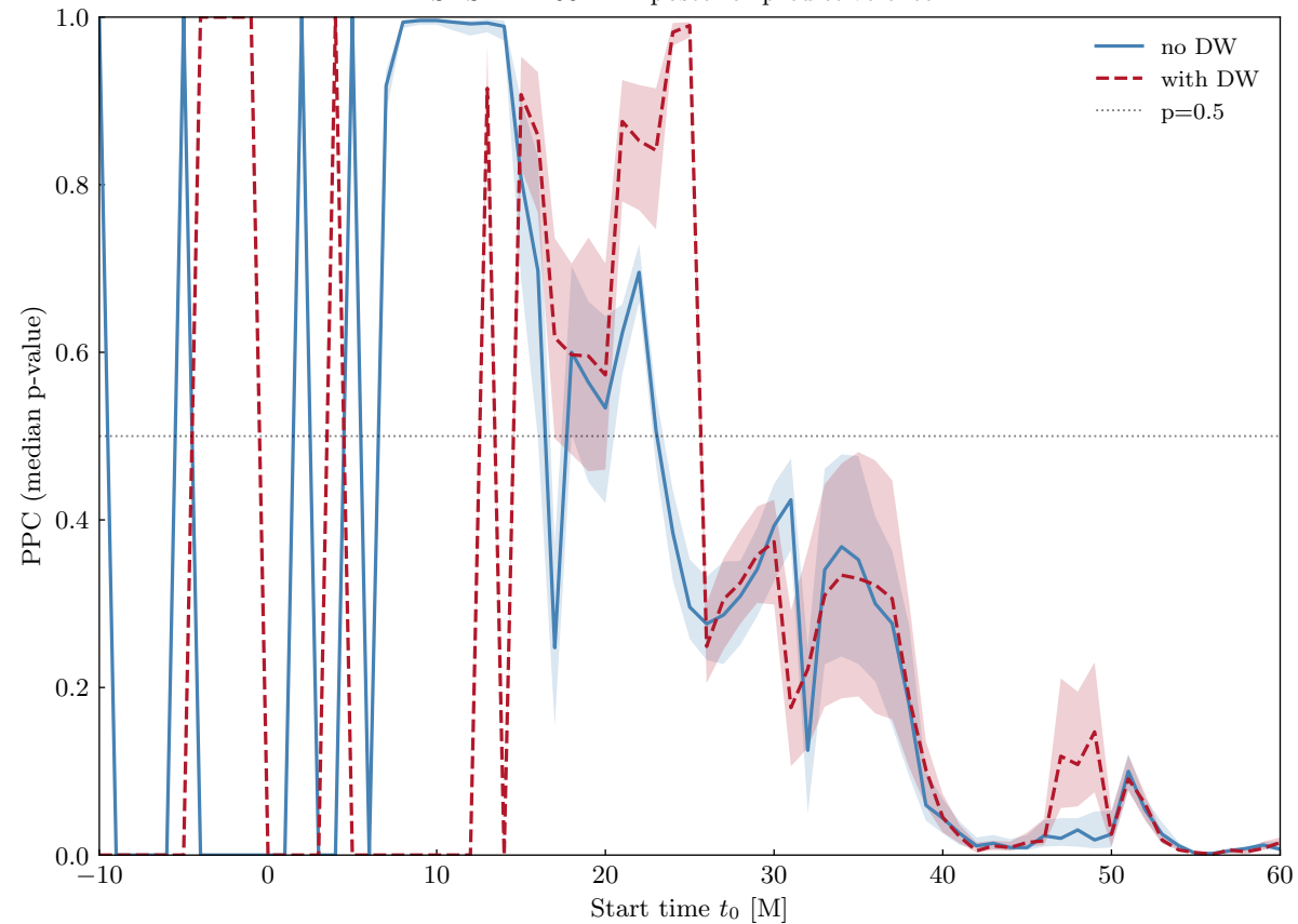
SXS:BBH:0012 — posterior predictive check
