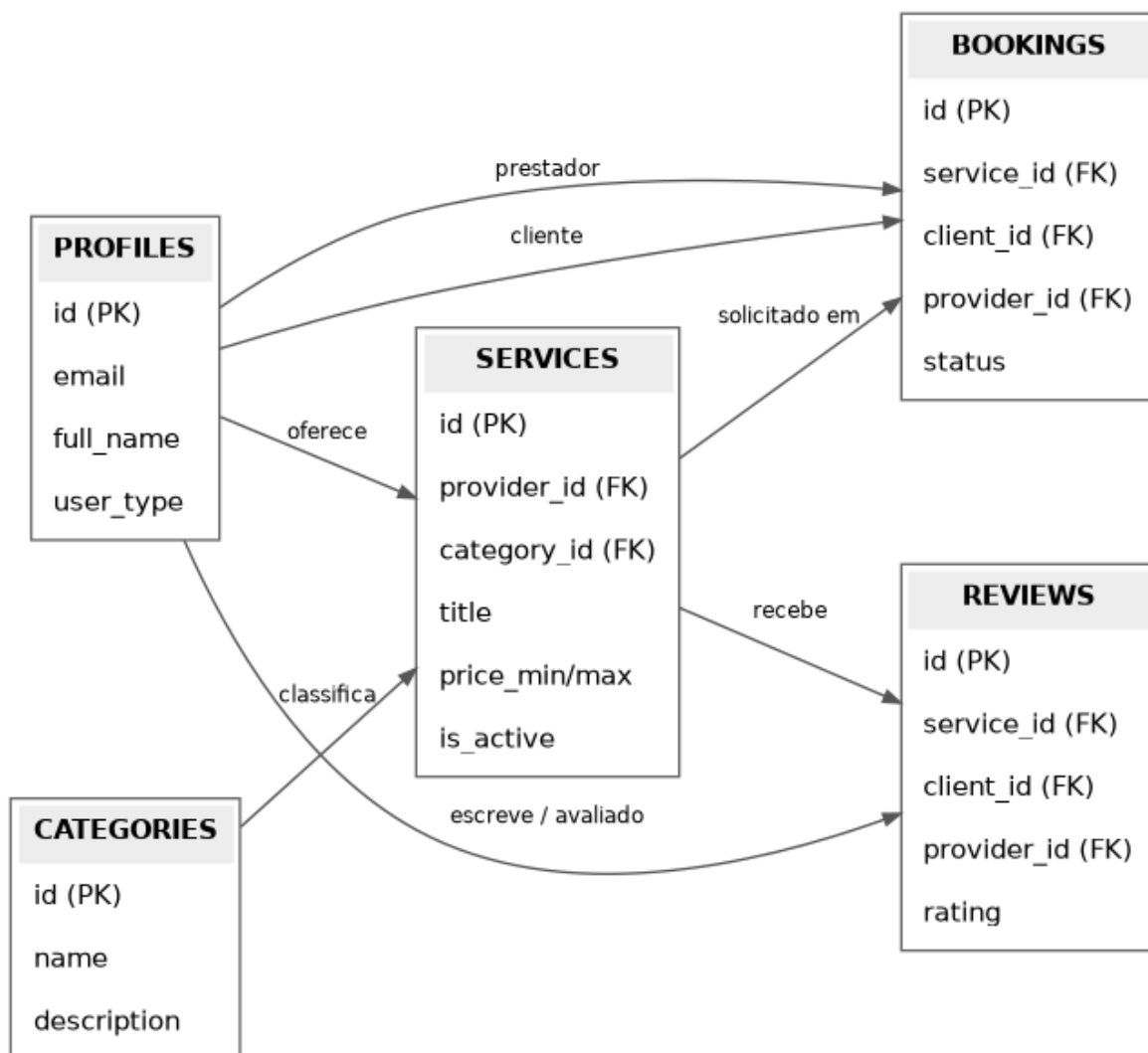
Figura A.1 — Diagrama Entidade-Relacionamento (DER)
