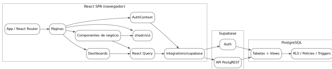
Figura A.7 — Diagrama de Componentes
