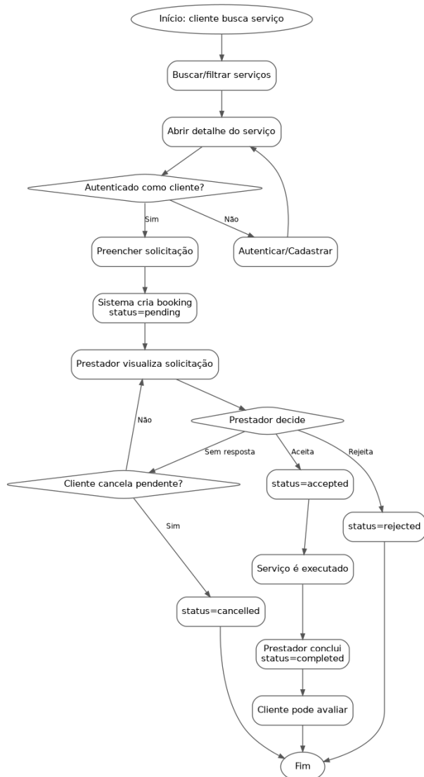
Figura A.9 — BPMN — Contratação de serviço
