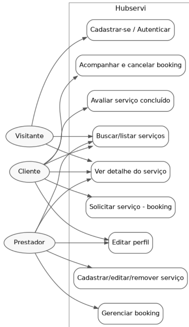
Figura A.2 — Diagrama de Casos de Uso
