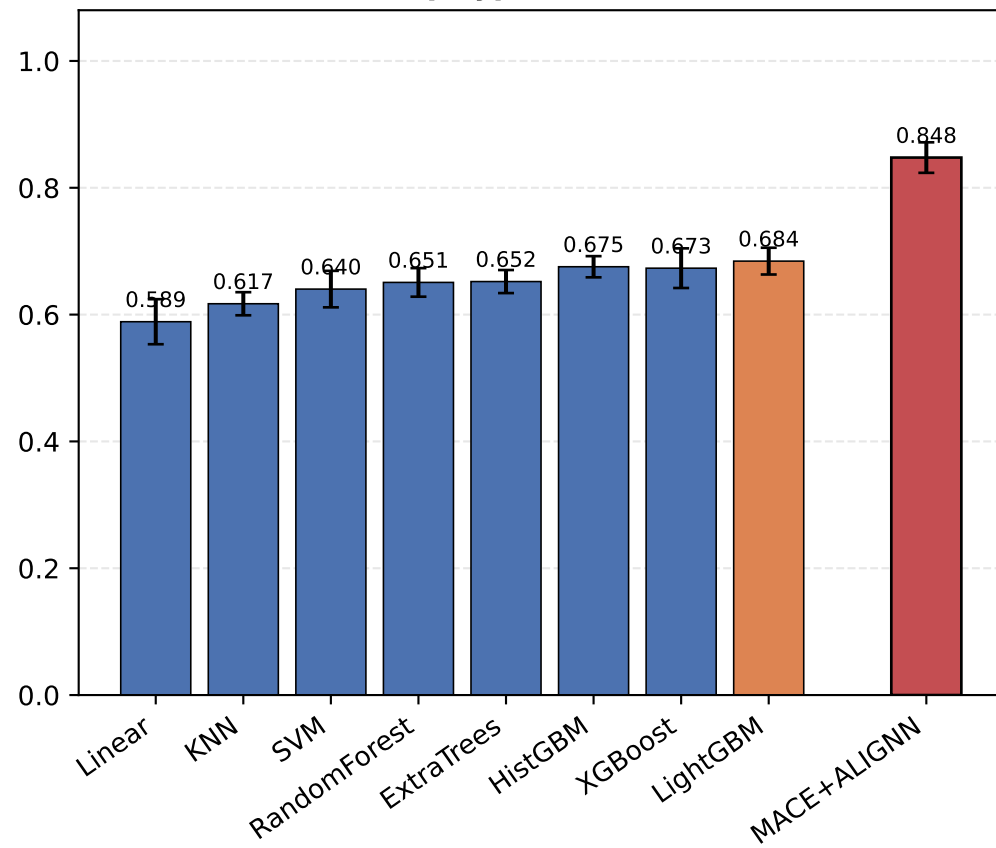
Gap-type macro-F1
