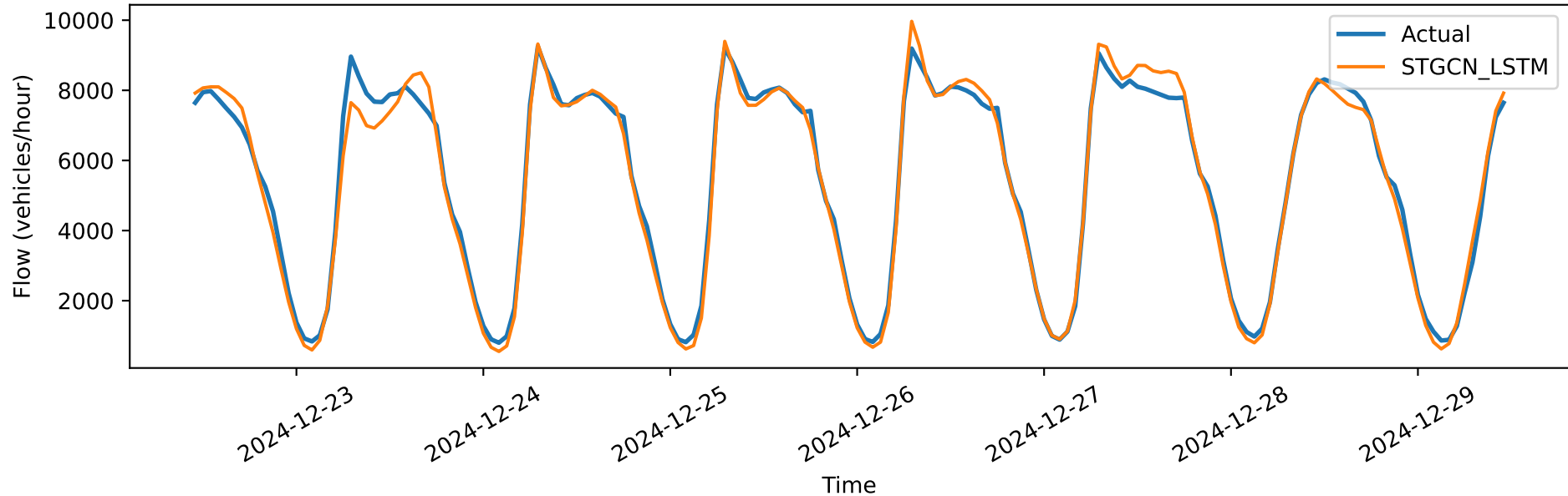
STGCN_LSTM vs Actual — 12h horizon — station 3015021
