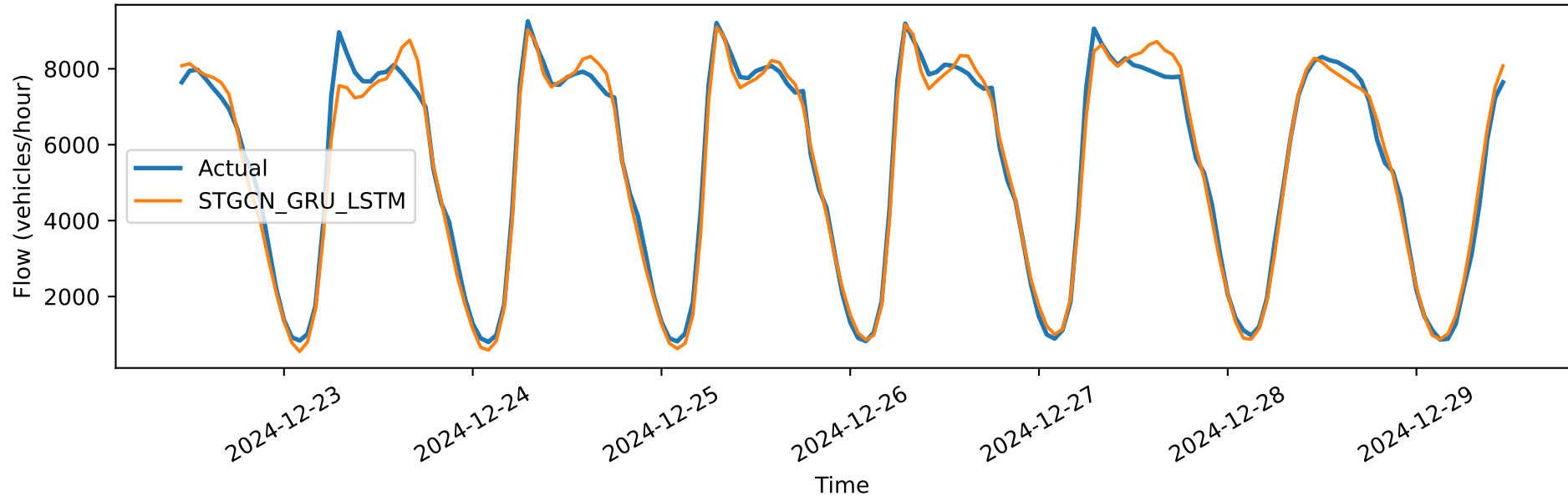
STGCN_GRU_LSTM vs Actual — 12h horizon — station 3015021
