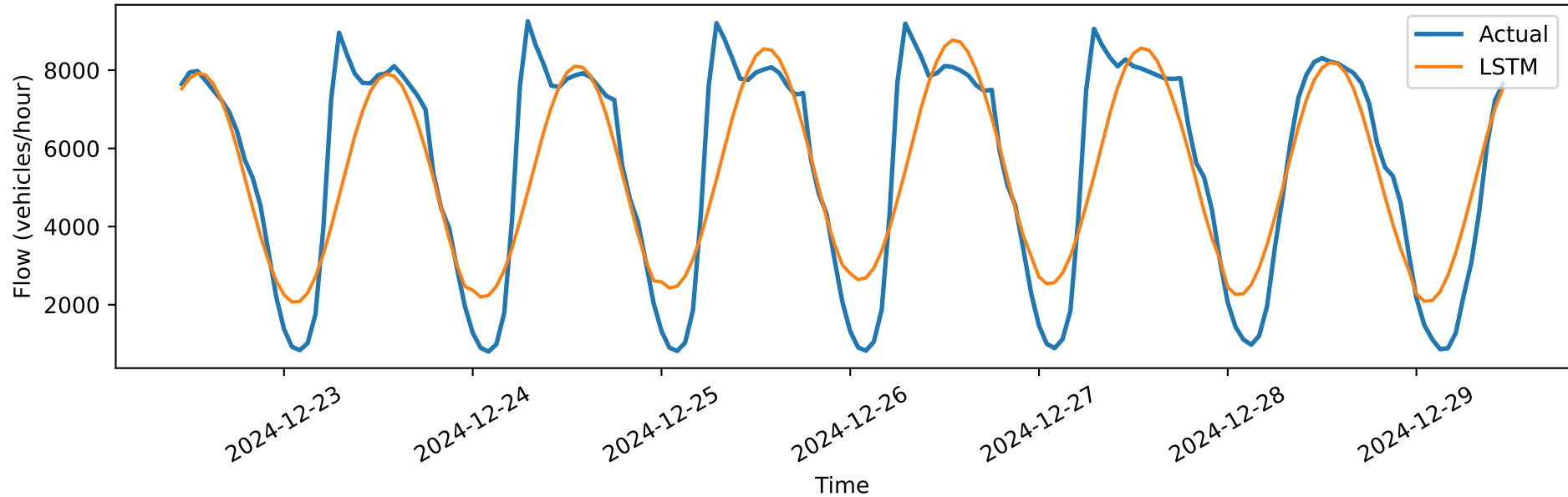
LSTM vs Actual — 12h horizon — station 3015021
