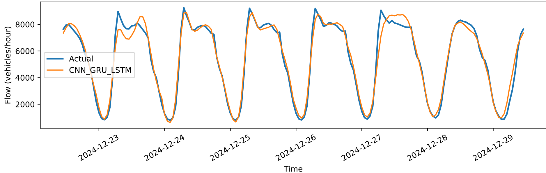
CNN_GRU_LSTM vs Actual — 12h horizon — station 3015021
