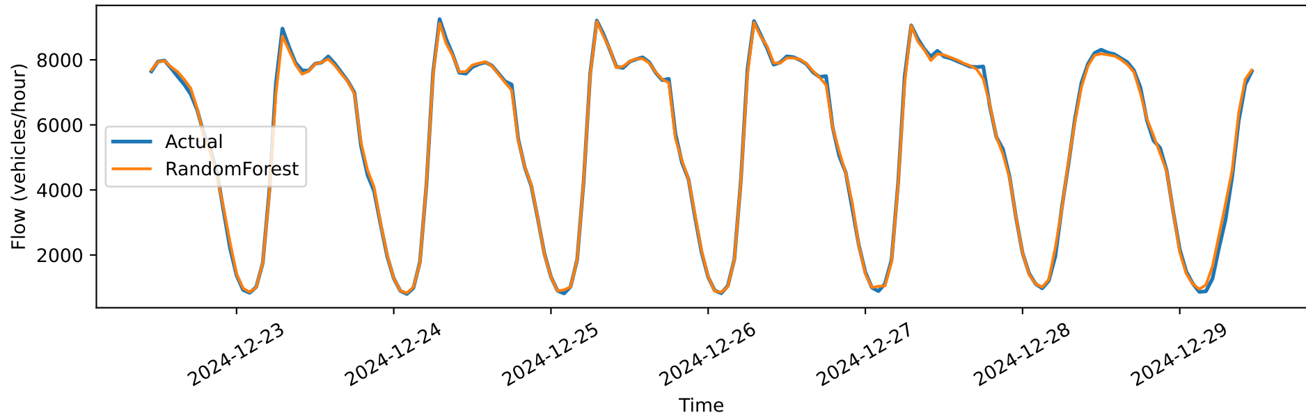
RandomForest vs Actual — 12h horizon — station 3015021
