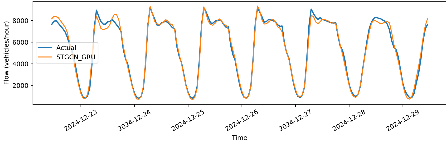
STGCN_GRU vs Actual — 12h horizon — station 3015021
