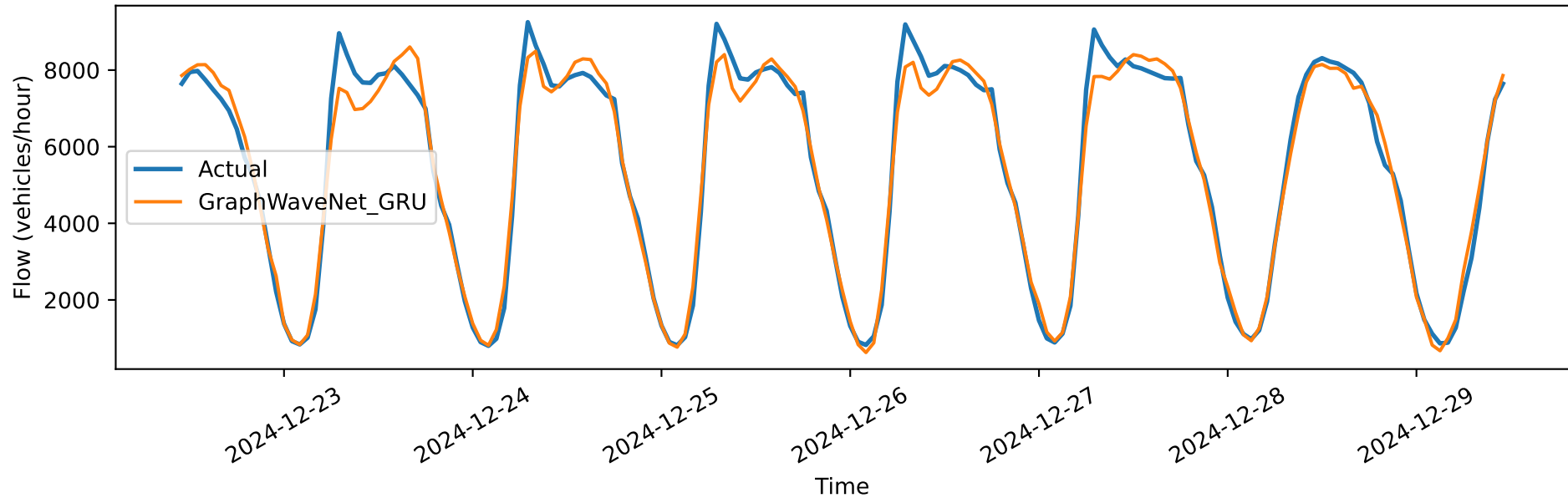
GraphWaveNet_GRU vs Actual — 12h horizon — station 3015021
