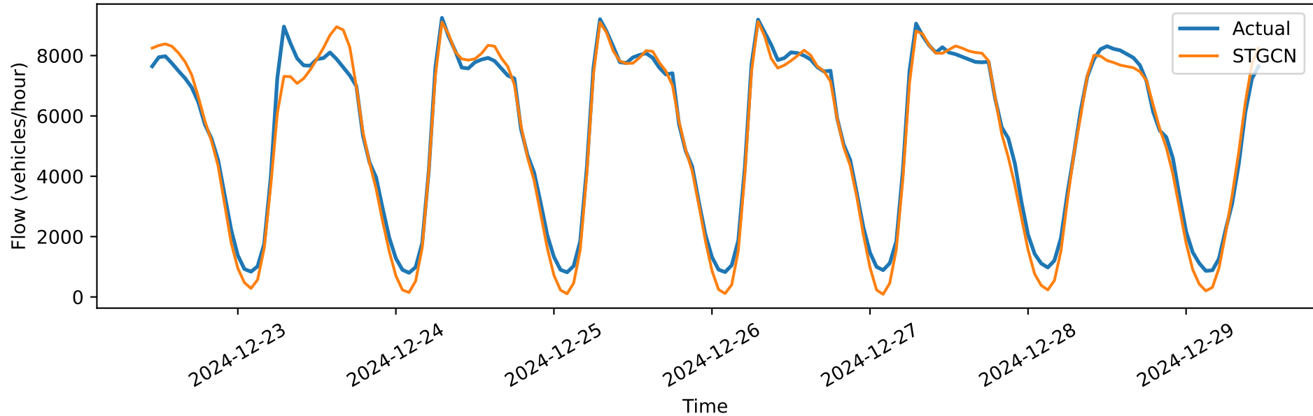
STGCN vs Actual — 12h horizon — station 3015021
