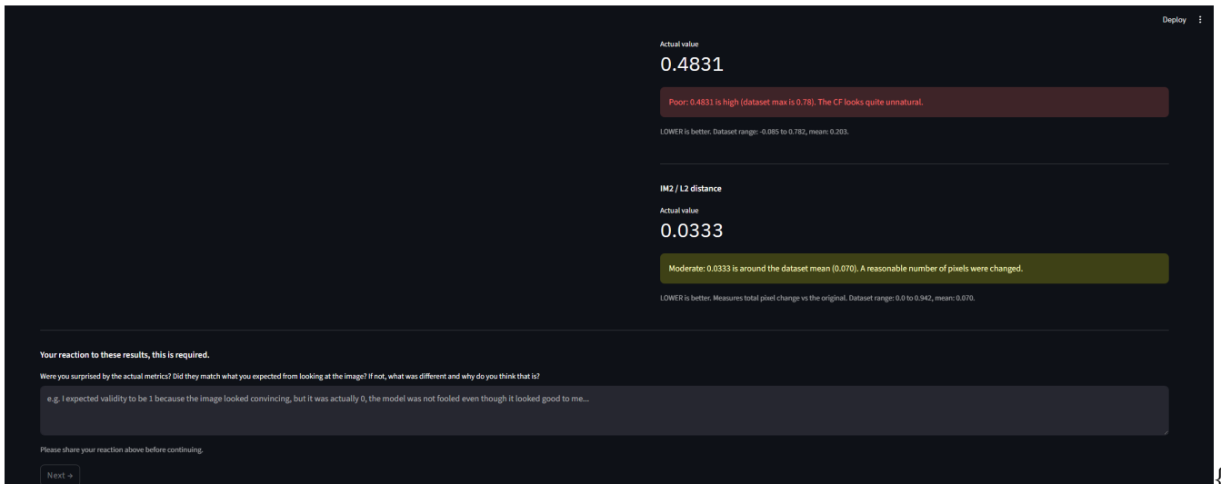
Figure 15: Actual metric 2
