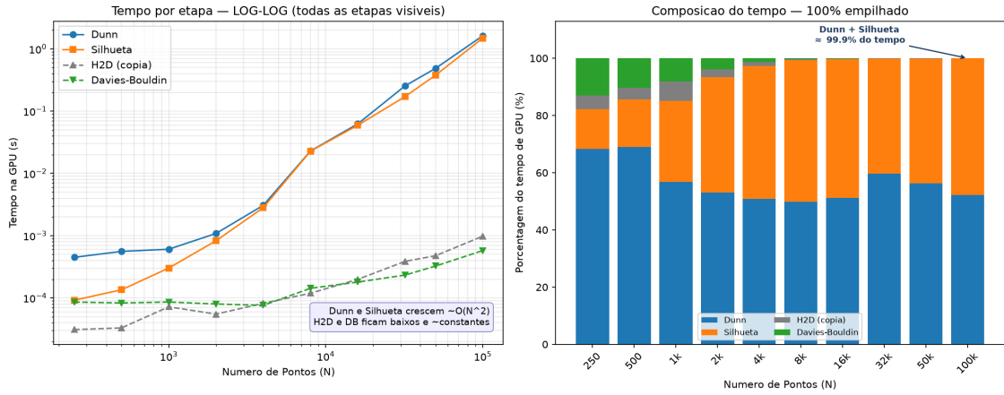
Figura 3. Decomposição do tempo de GPU por etapa. Esquerda: escala log-log (todas as etapas visíveis). Direita: composição percentual.
