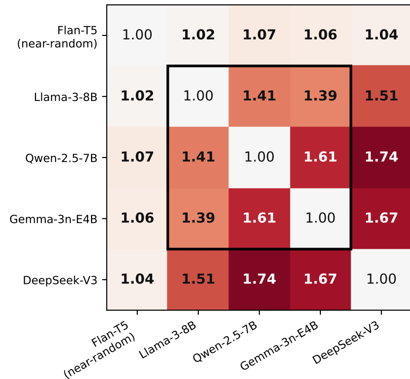
MedQA-USMLE
