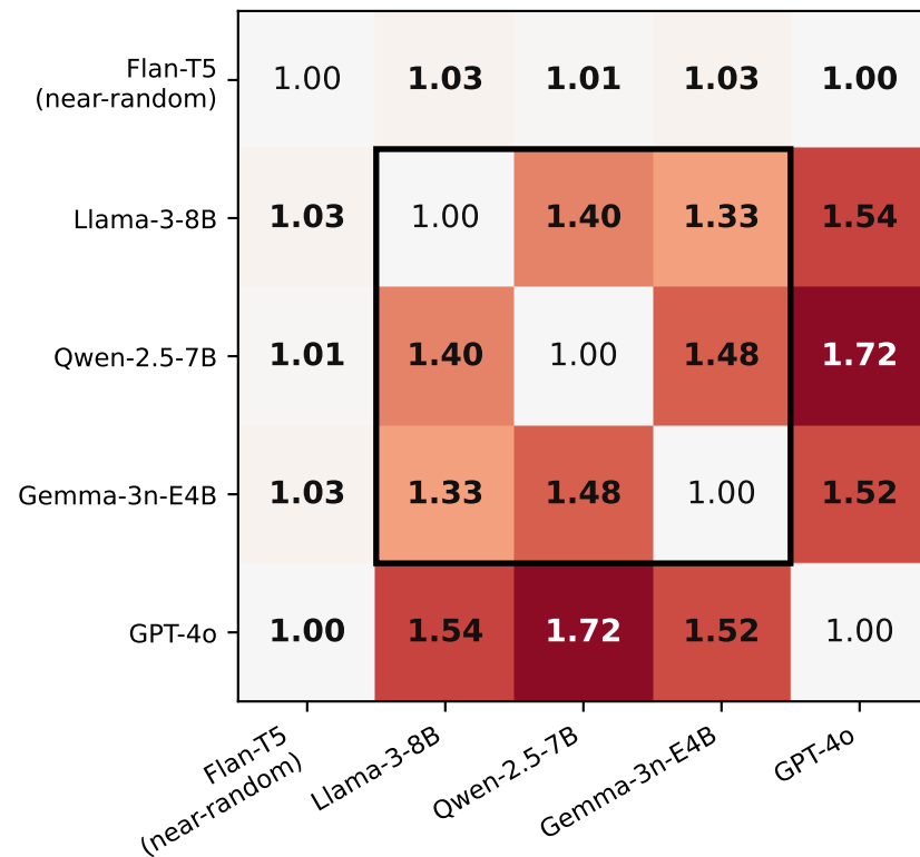
MedMCQA
