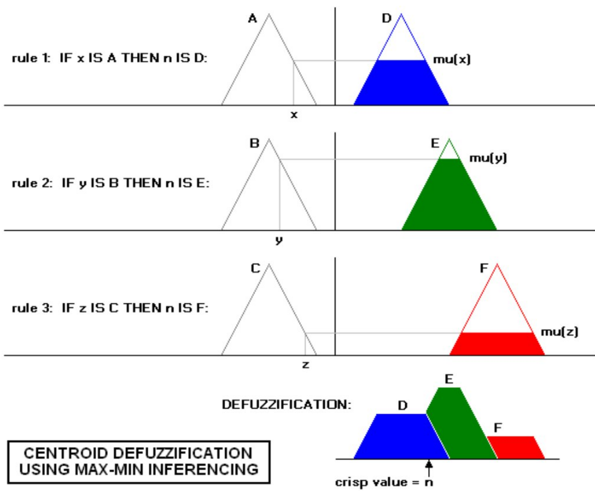
9 Ábra: Defuzzifikáció
