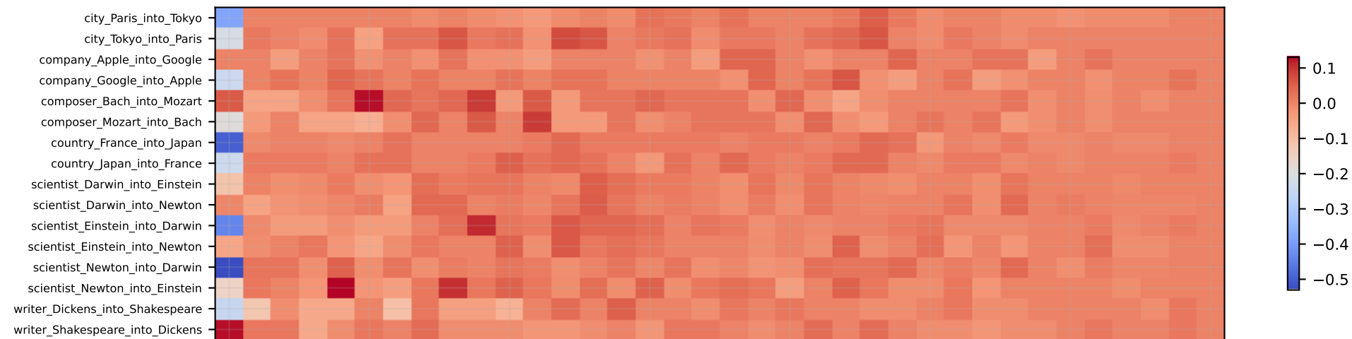
MLP effect P02
