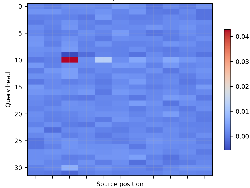
Layer 23
