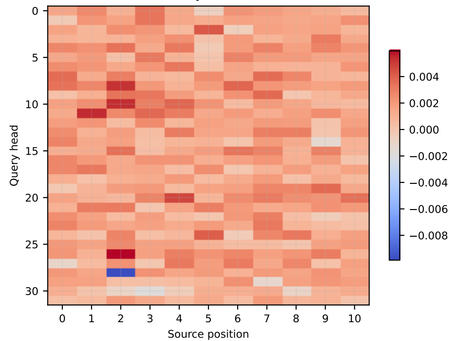
Layer 25
