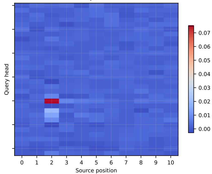
Layer 26
