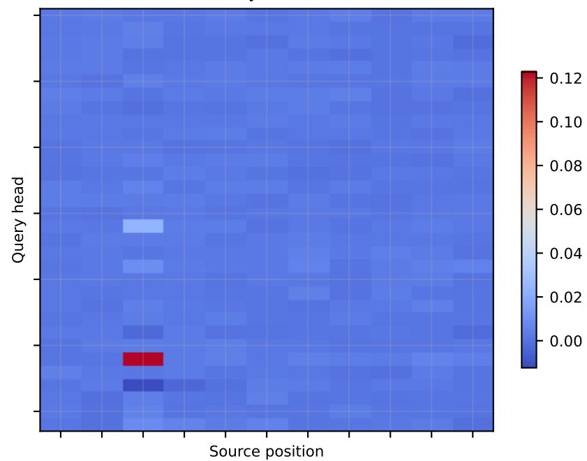
Layer 24
