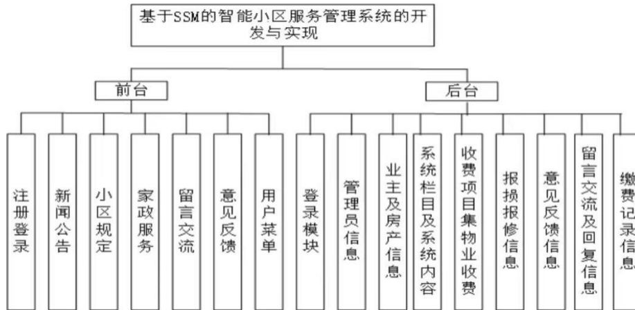
图 5-1 系统总体功能结构图
