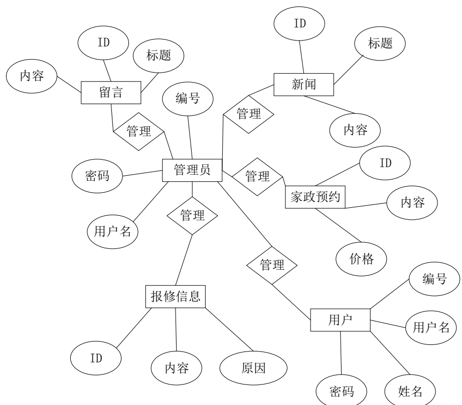
图 5-6 管理员 E-R 图
