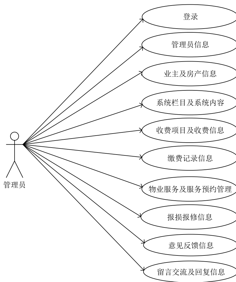
图 4-2 后台管理员用例图
