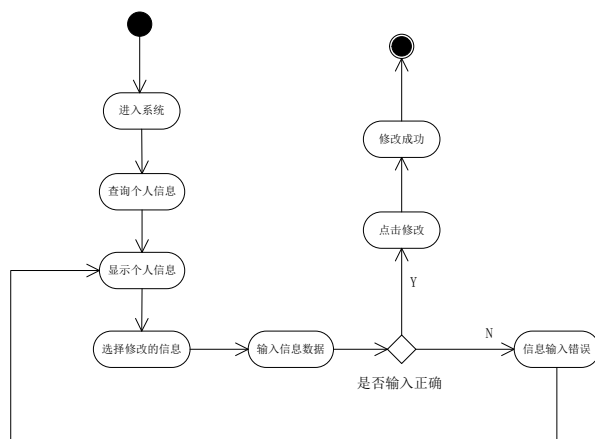
图 4-4 信息管理模块活动图
