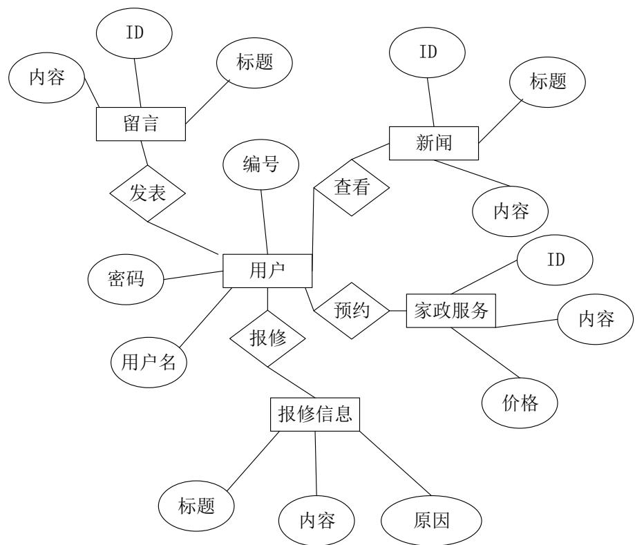
图 5-4 用户 E-R 图
