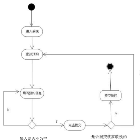
图 4-5 用户家政服务预约活动图
