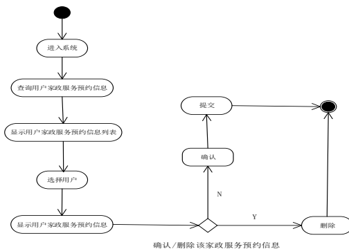
图 4-6 管理员家政服务预约管理活动图
