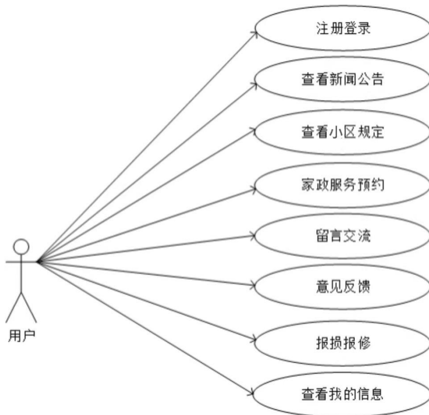
图 4-1 用户用例图
