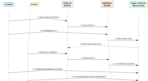
Fig. 2. Sequence diagram interaksi UI-wallet-contract untuk persetujuan milestone.
