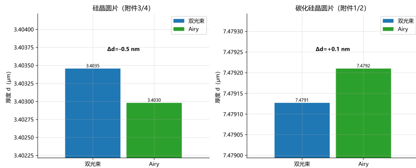
图 25 双光束与 Airy 模型的厚度结果对比
