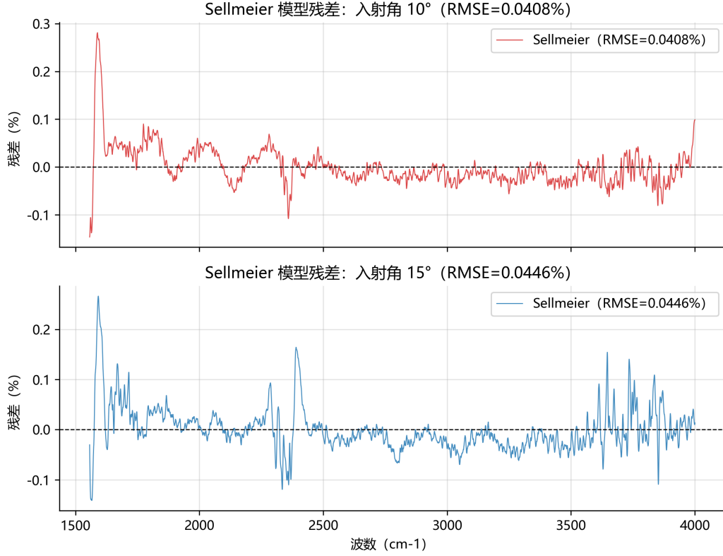
图 10 Sellmeier 单振子模型残差随波数的分布
