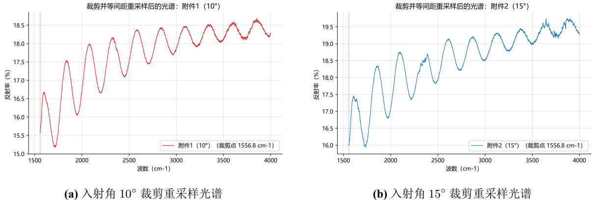
图 4 裁剪并等间距重采样后的反射率光谱
