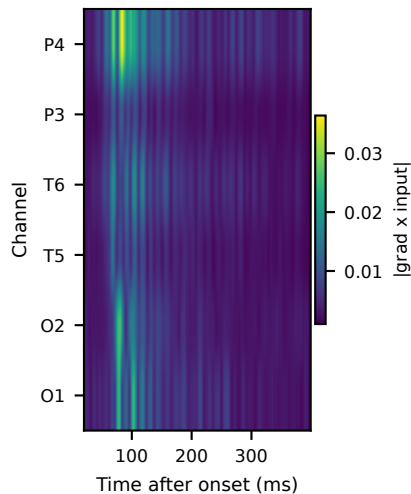
(d) Temporal saliency
