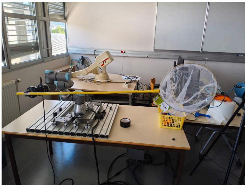
FIGURE 8.1 – Montage réel avec robot, caméra et zone de réception.
