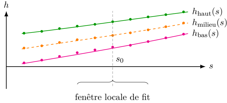
FIGURE 5.5 – Les trois courbes du ruban sont ajustées à partir des échantillons valides. L’ajustement est local : autour de s_0 , les points proches pèsent davantage que les points éloignés.
