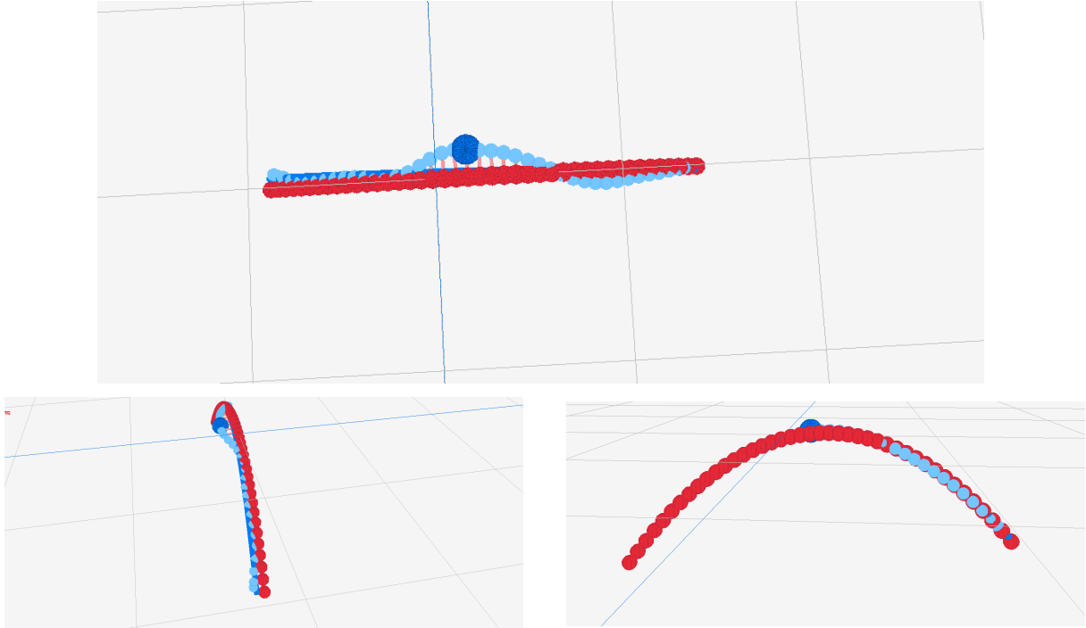
FIGURE 6.2 – Sorties 3D obtenues avec la méthode Trace. Chaque carré de la grille correspond à 25 cm. Les points bleus sont les estimations de l'algorithme et les points rouges sont les positions réelles issues d'Isaac Sim [9].
