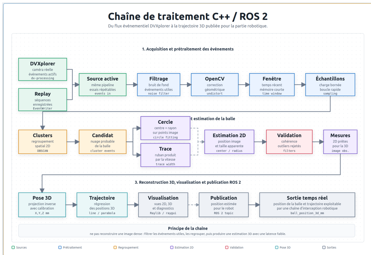
FIGURE 3.1 – Chaîne de traitement C++/ROS 2 [6] utilisée pour l'estimation 3D de la balle.
