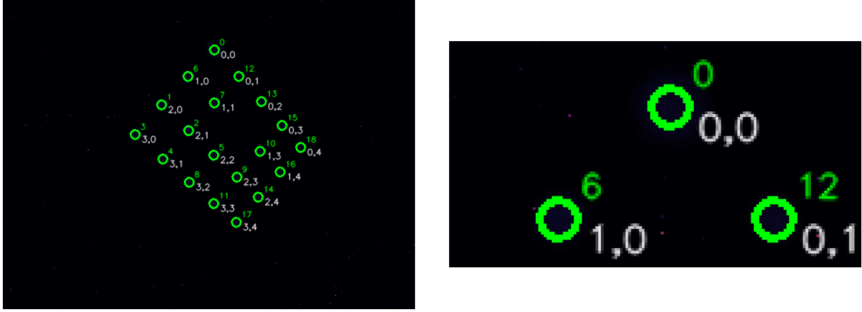
FIGURE 7.4 – Exemple de sortie de l'algorithme de détection de la mire événementielle. L'écran est décalé et n'est pas face à la caméra ; à droite, la vue zoomée met mieux en évidence les événements. La couleur des événements correspond à un choix provisoire de visualisation qui n'a pas été modifié ensuite.
