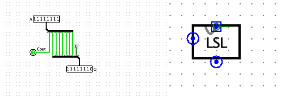
1.2. attēls LSL operācija.
