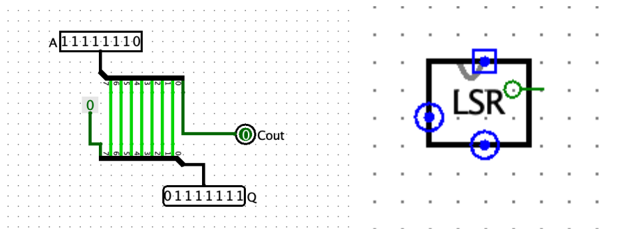
1.3. attēls LSR operācija.
