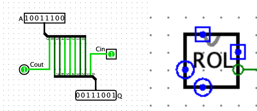
1.4. attēls ROL operācija.
