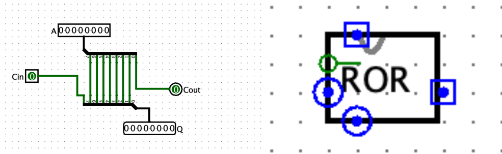
1.5. attēls ROR operācija.
