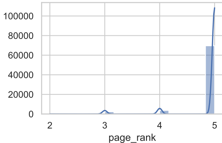
page_rank
