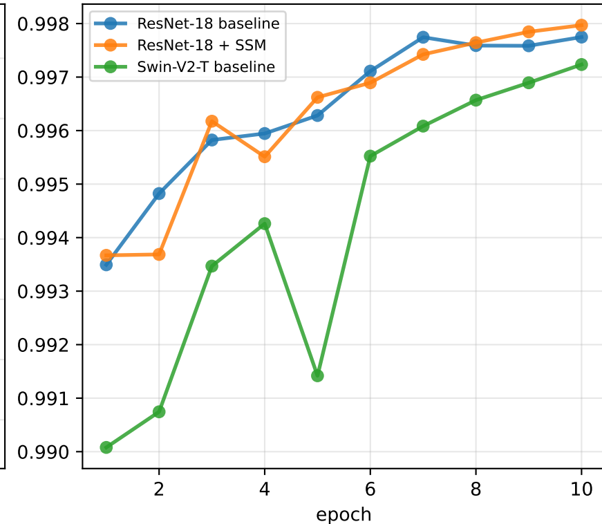
(d) Validation macro AUC
