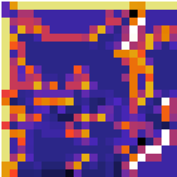
Pooling: axis1
