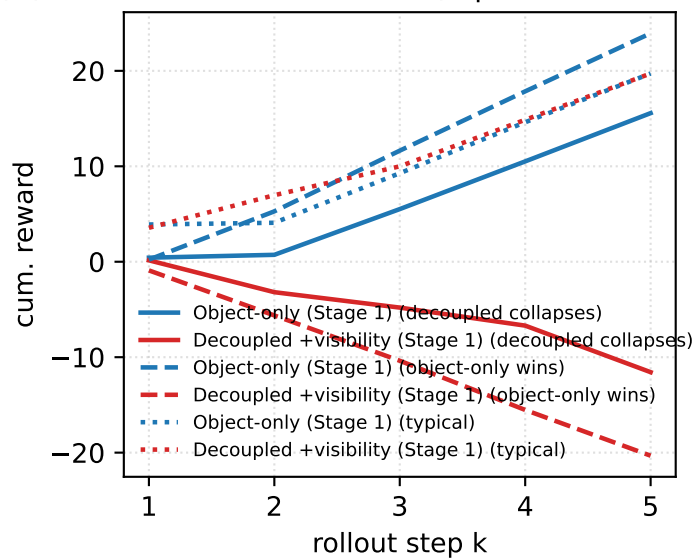
(D) Cumulative latent return (representative samples)
