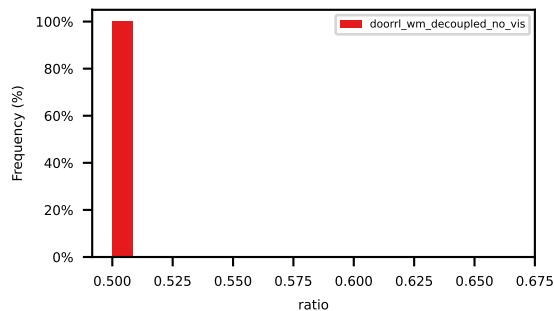
ratio_of_failed_ego_lane_change
