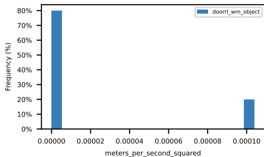
p90_ego_lat_acceleration
