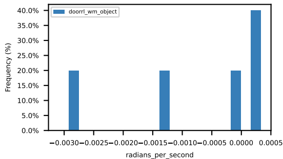
abs_ego_yaw_rate_within_bounds
