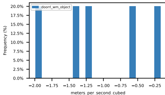
p90_ego_jerk
