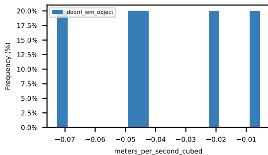
abs_ego_lon_jerk_within_bounds
