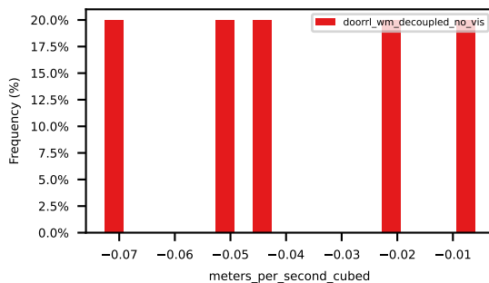
abs_ego_jerk_within_bounds
