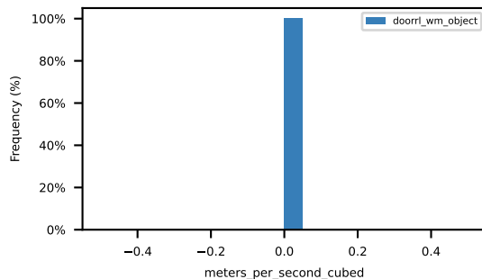
avg_ego_jerk
