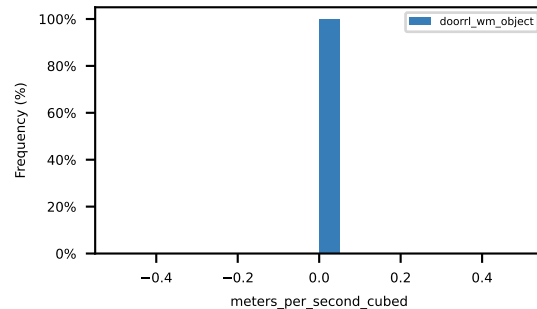
p90_ego_jerk
