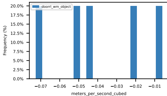
abs_ego_jerk_within_bounds
