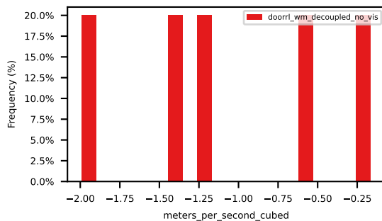
p90_ego_jerk
