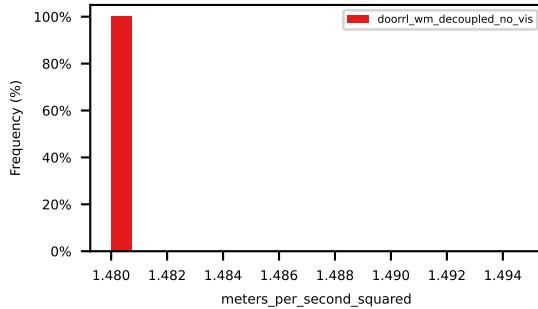
avg_ego_lon_acceleration
