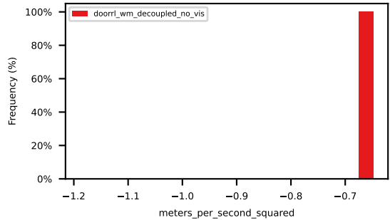
p90_ego_lon_acceleration
