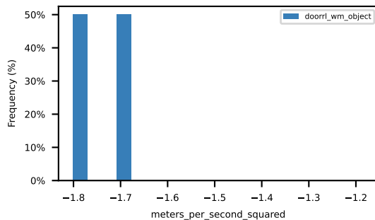
p90_ego_lon_acceleration
