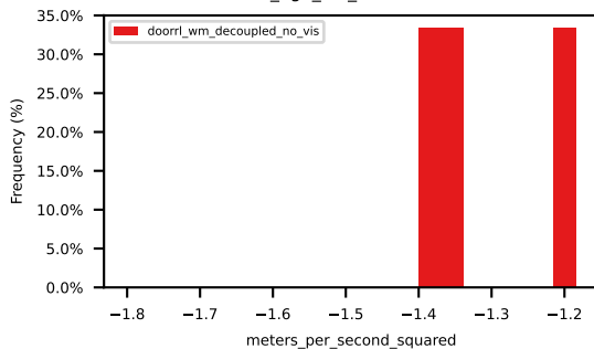
p90_ego_lon_acceleration
