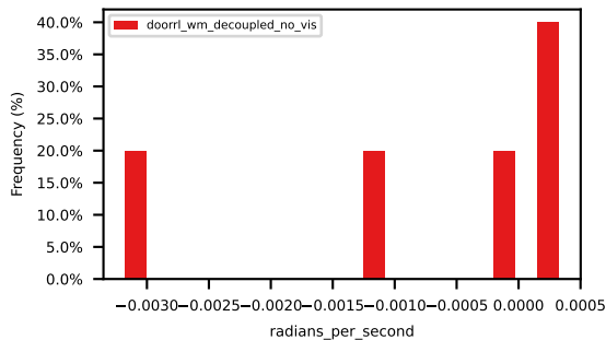
abs_ego_yaw_rate_within_bounds
