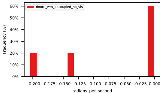
abs_ego_yaw_rate_within_bounds
