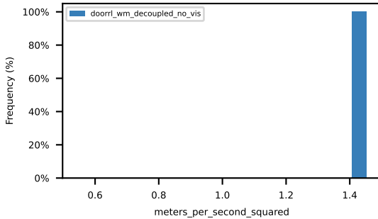
avg_ego_lon_acceleration
