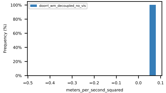
p90_ego_lon_acceleration
