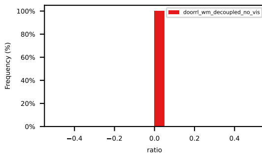
ratio_of_failed_ego_lane_change
