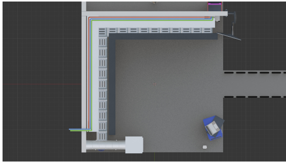
Figura 3.14: Vista de Viewport do caminho de cabos (Vista de cima).
