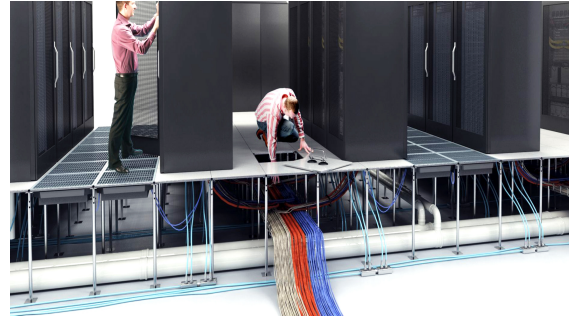
Figura 3.11: Ilustração do pavimento técnico.
