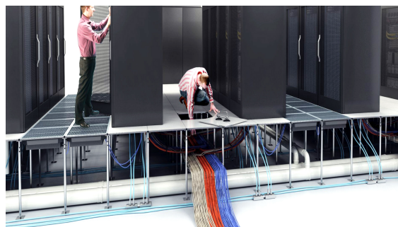
Figura 3.12: Ilustração do pavimento técnico.
