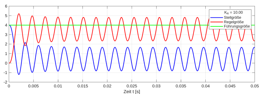
6 Abbildung 2: Matlab -Plots für verschiedene Reglerverstärkungen
