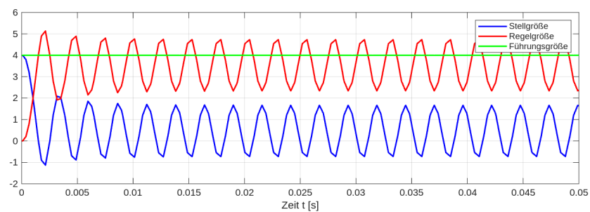
6 Abbildung 2: Matlab -Plots für verschiedene Reglerverstärkungen
