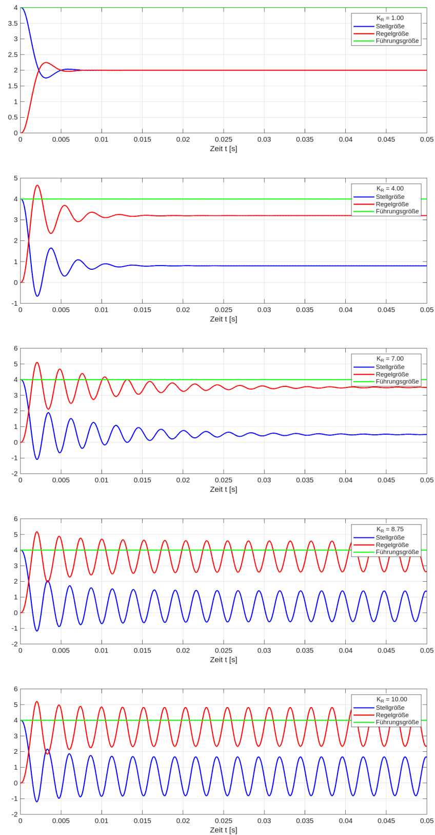
Abbildung 2: Matlab -Plots für verschiedene Reglerverstärkungen
