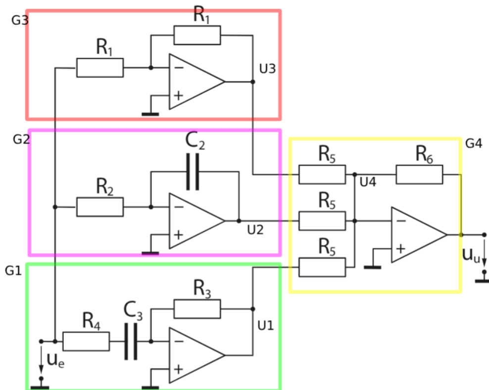
Abbildung 6: Elektronischer Aufbau des PID-Reglers (Screenshot aus der Aufgabenstellung)
