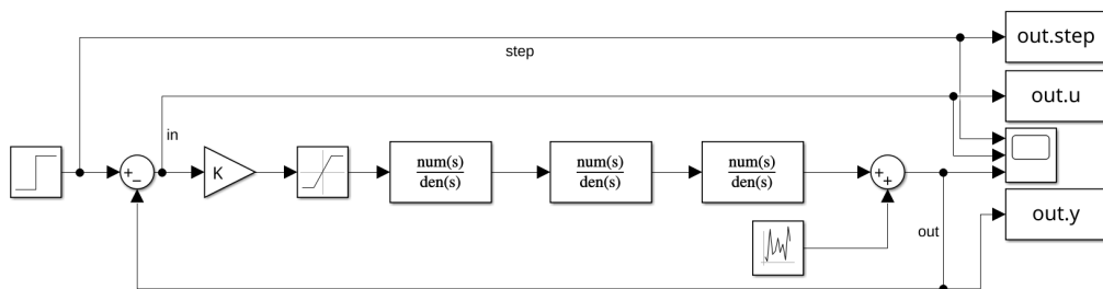
Abbildung 4: Blockschaltbild (Screenshot aus Simulink )
