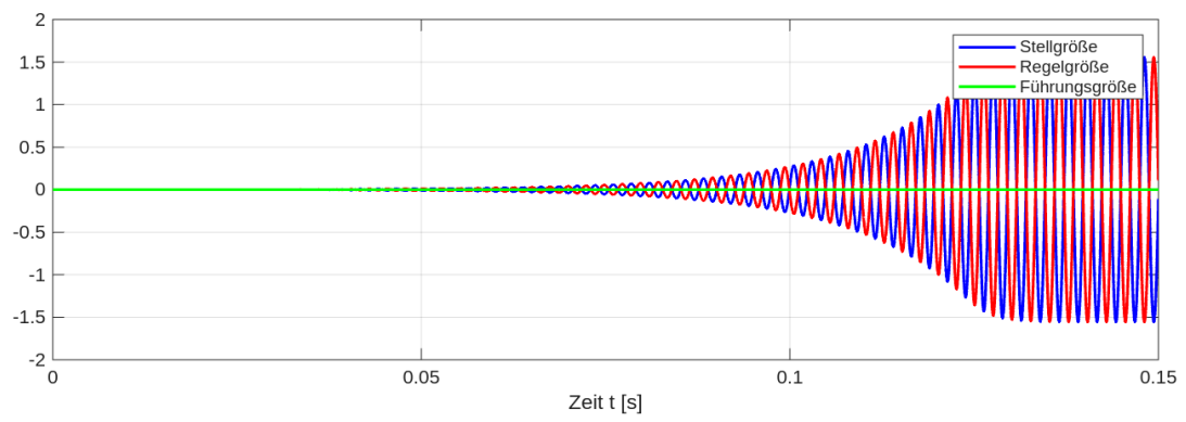
Abbildung 5: Matlab -Plot für w(t) = 0 (mit Rauschquelle)
