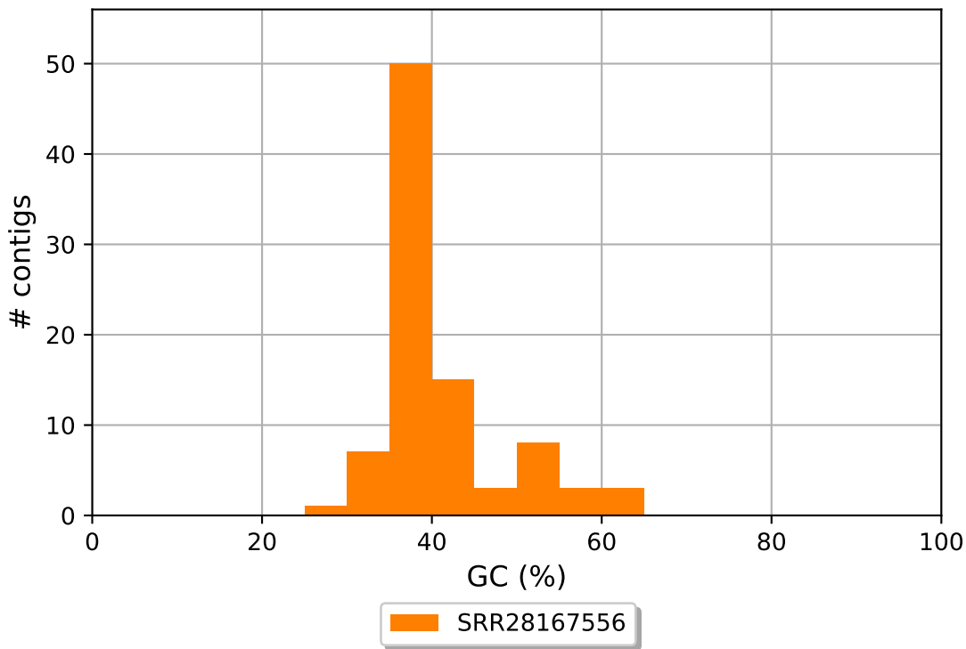
SRR28167556 GC content
