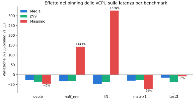
Fig. 39. Effetto del pinning delle vCPU sulla latenza per benchmark
