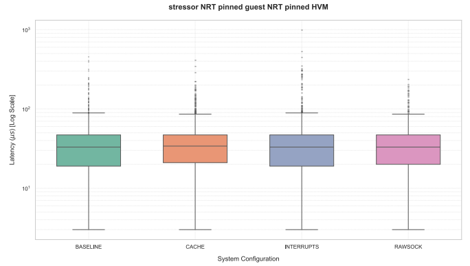
Fig. 25. stressor on Xen
