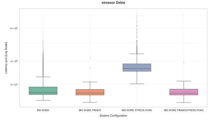
Fig. 40. TACLe benchmark - debie stress dom0
