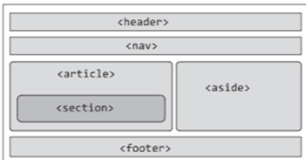
Рис. 1.12. Задание структуры страницы на языке HTML5 с помощью новых структурных элементов
