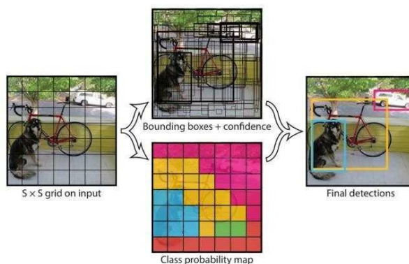
รูปที่ 2.11 หลักการทำงานของ YOLO
