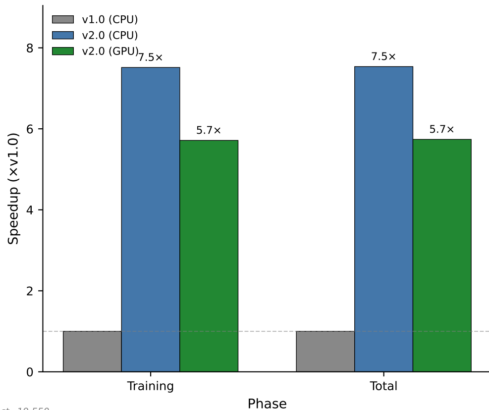
Dataset: Bassez
