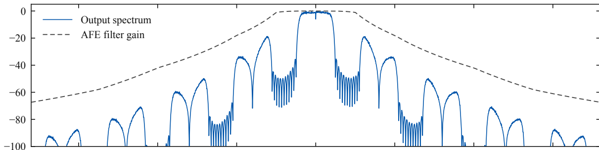
(b) 2 sps, filter tune 4 + EQ
