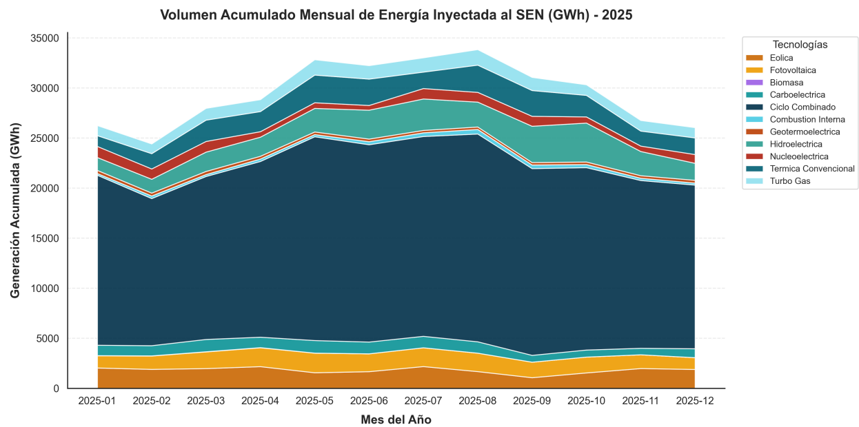
Figura 4: Volumen acumulado mensual (Área apilada en GWh).
