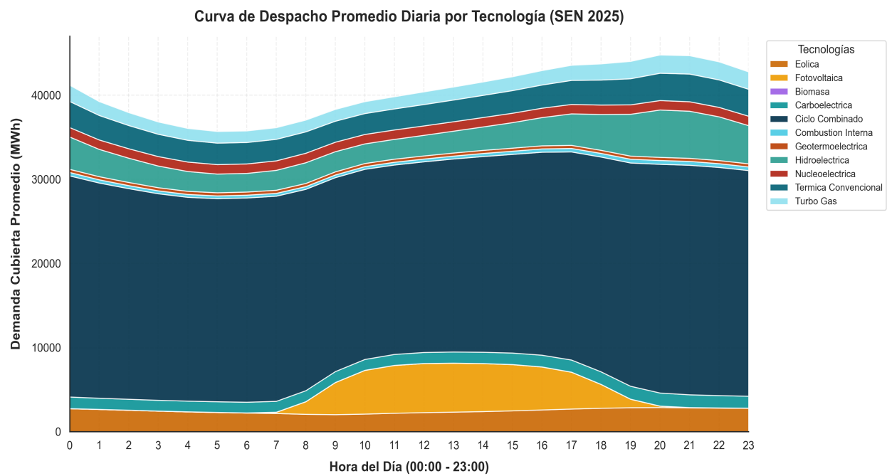
Figura 5: Curva de despacho horaria promedio (Interacción tecnológica 00:00 - 23:00).
