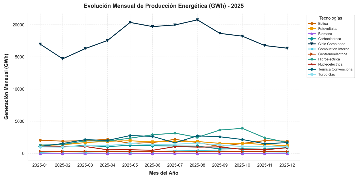
Figura 3: Evolución mensual por tecnología en GWh.
