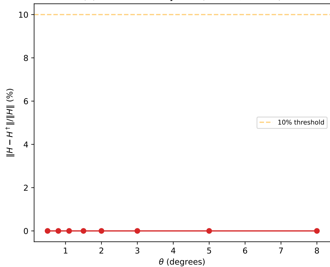
(d) Non-Hermiticity of H (Band 1, N_s=32 )
