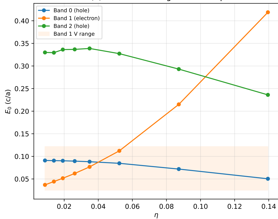
(d) Ground state eigenvalue vs \eta
