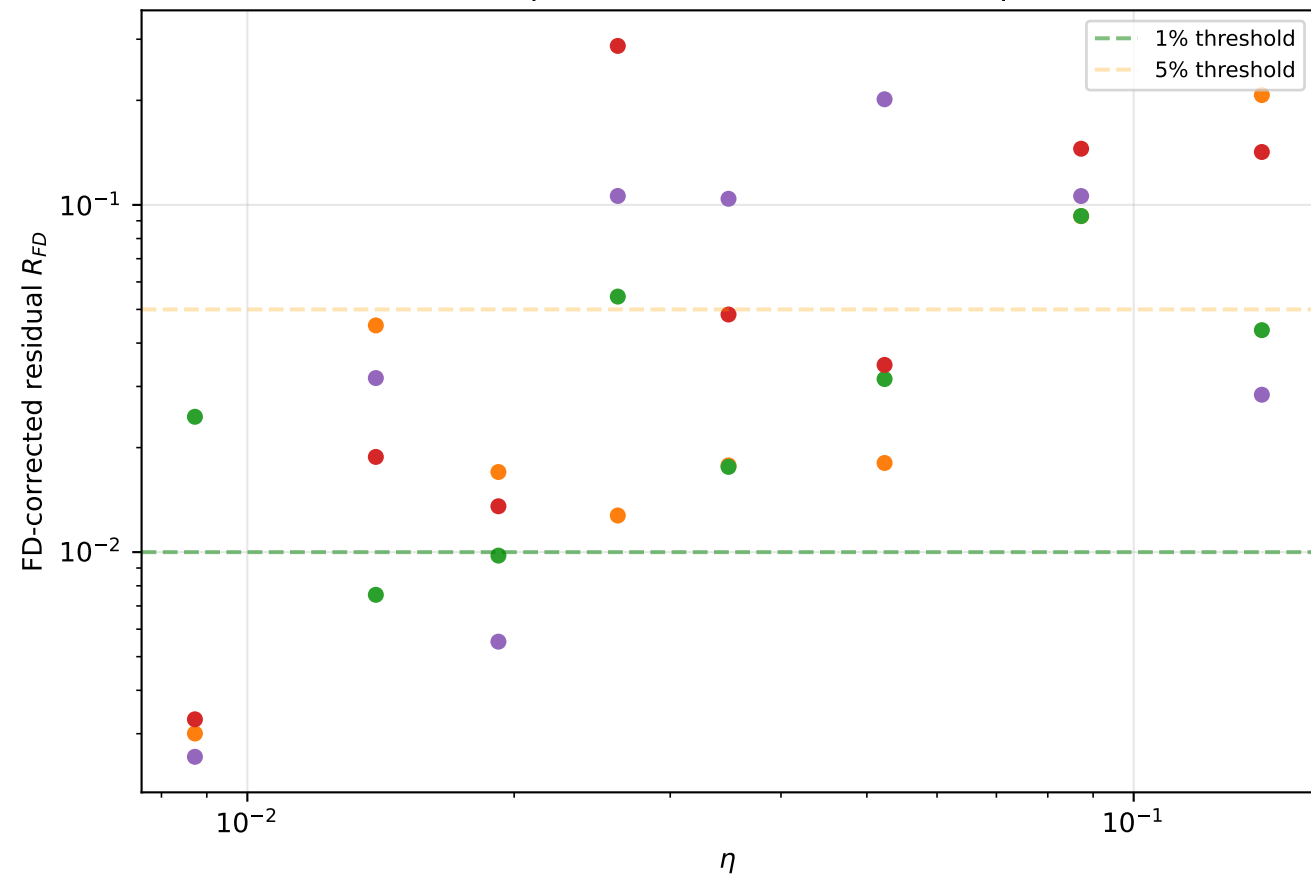
(d) Option C: Maxwell residual vs η
