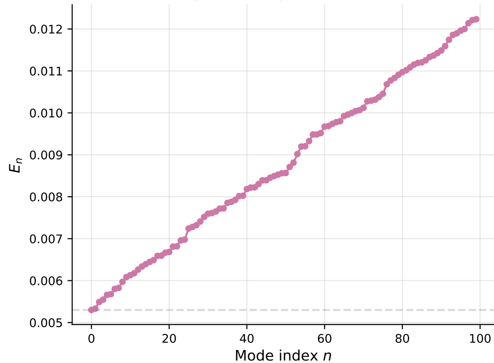
(a) Eigenvalue spectrum (N=100)
