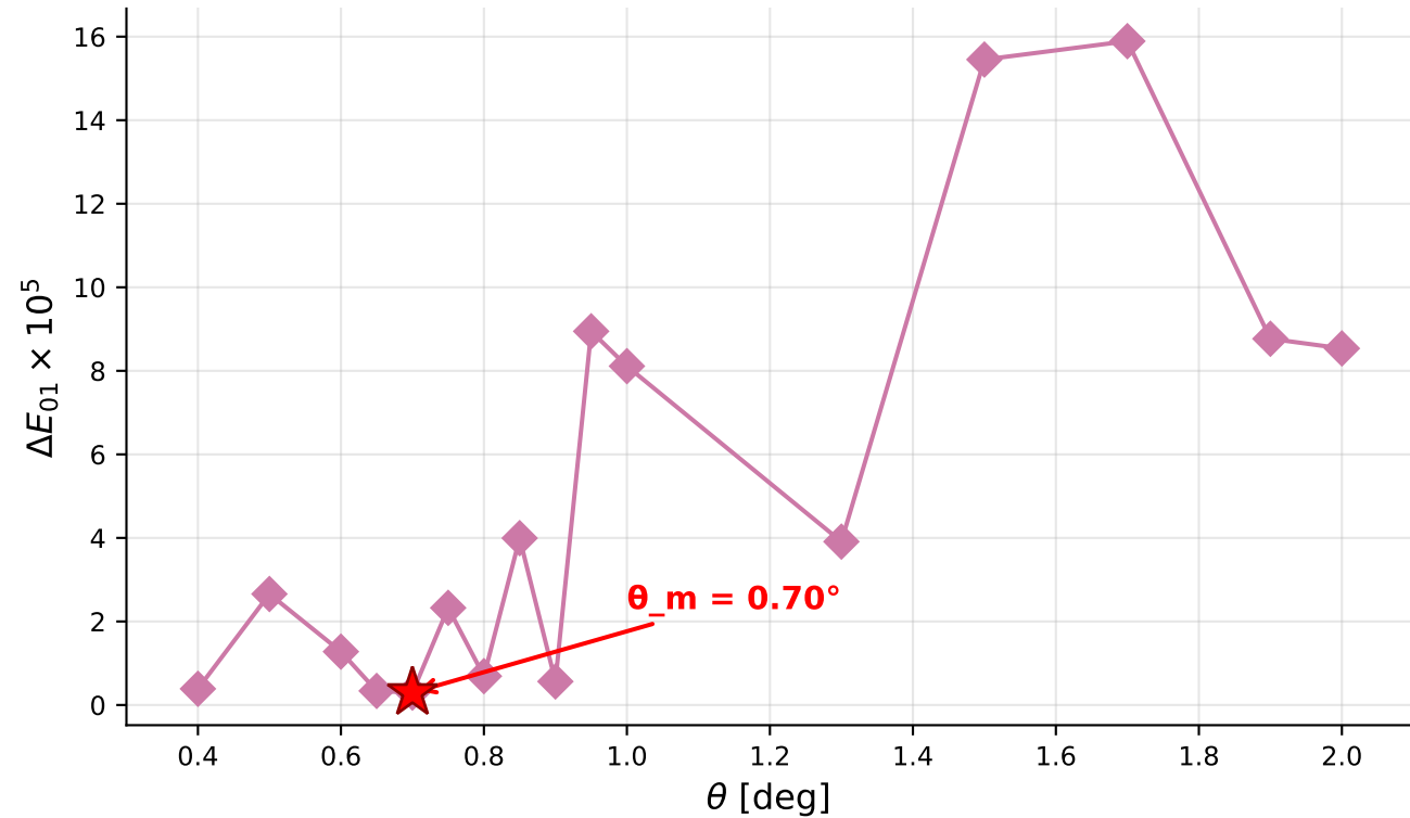
(a) Fine gap structure (linear scale)
