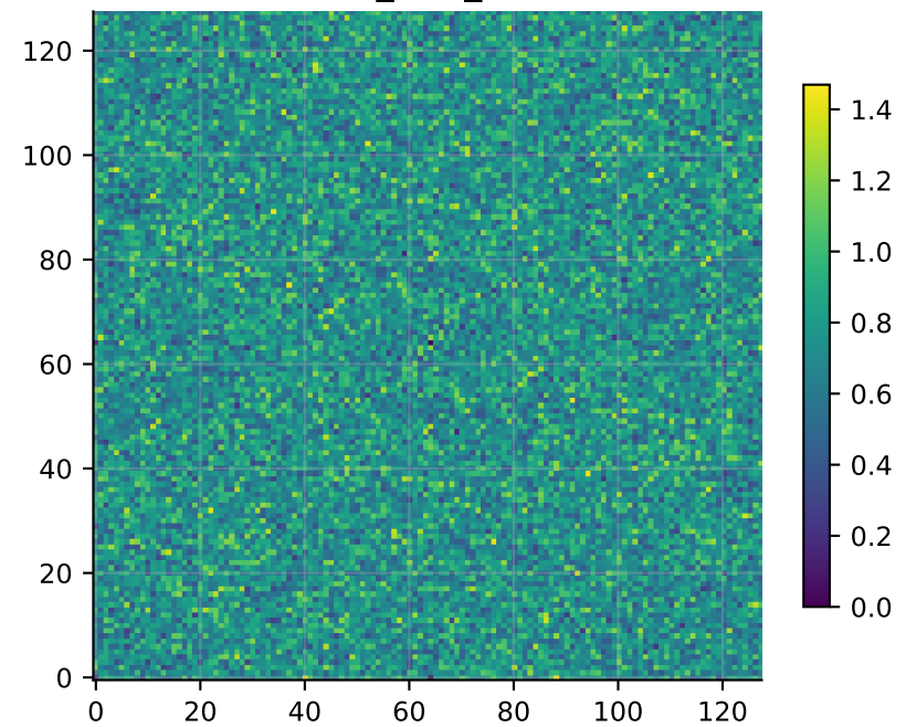
A_{\text{frob}_x}
