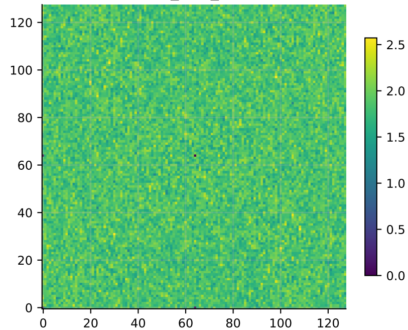
A_frob_y
