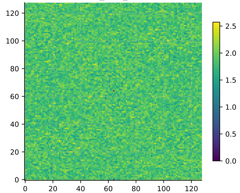
A_frob_x
