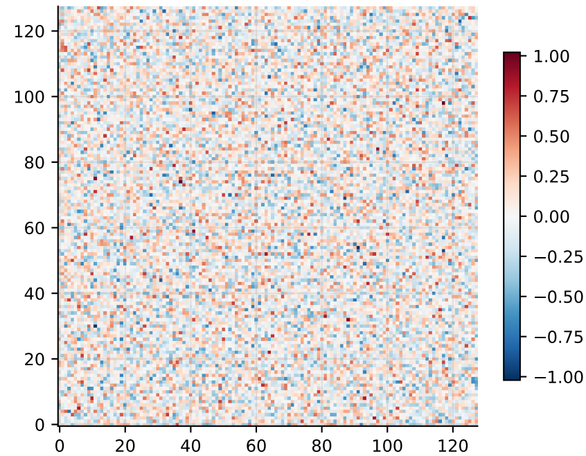
A_frob_y
