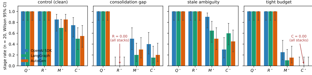
Рис. 5: Постадийные профили трёх сторонних агентных стеков на четырёх инженерных вариантах (Папа3.1, n=20 на ячейку). Запрос и извлечение насыщаются везде идентично; два структурных отказа дают точные нулевые столбцы на каждом стеке ( R^*=0 при консолидационном разрыве, C^*=0 при жёстком бюджете); поведенческий разброс между фреймворками целиком живёт на стадиях М и С.
