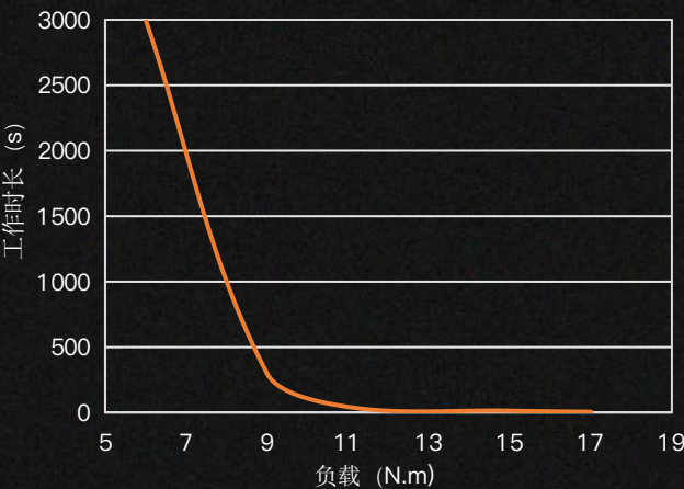
堵转工况最大过载曲线 ( Max Overload )
