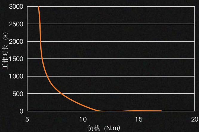
堵转工况最大过载曲线 ( Max Overload )
