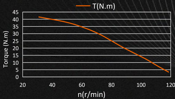
48V T-N曲线 (T-N under 48V)
