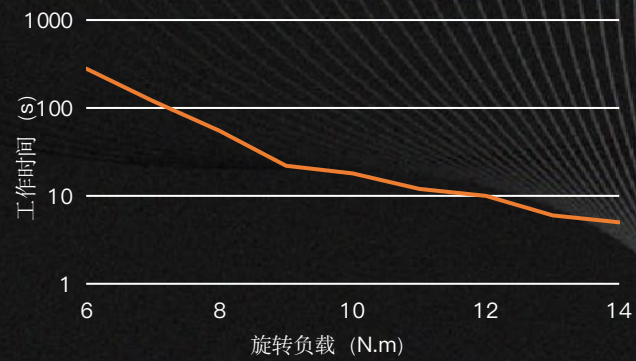
堵 转 工 况 最 大 过 载 曲 线 ( Max Overload )
