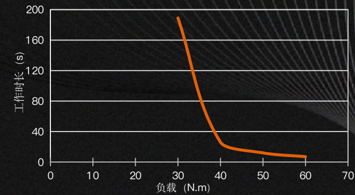
旋转工况最大过载曲线 ( Max Overload ) ( 200mm×200mm铝散热板 )
