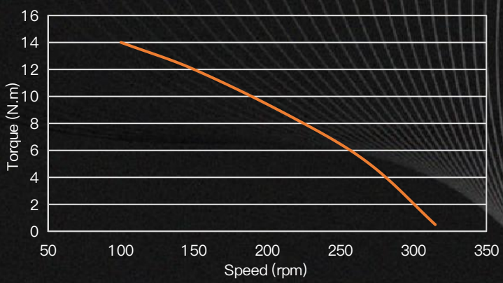
热平衡态T-N曲线 Thermal equilibrium state T-N curve ( 150mm×150mm铝散热板 )
