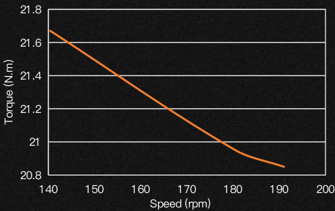
热平衡态T-N曲线 Thermal equilibrium state T-N curve ( 200mm×200mm铝散热板 )
