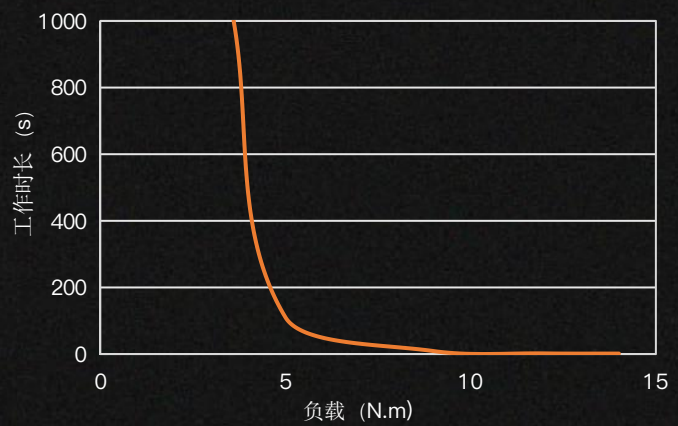
堵 转 工 况 最 大 过 载 曲 线 ( Max Overload )
