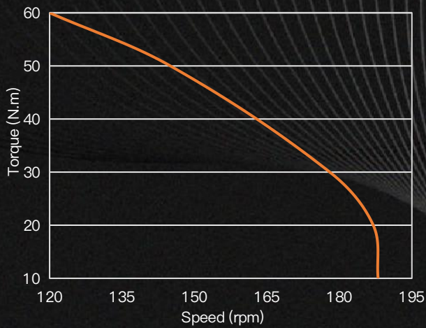
热平衡态T-N曲线 Thermal equilibrium state T-N curve ( 200mm×200mm铝散热板 )
