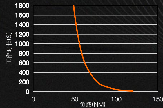
旋转工况最大过载曲线 ( Max Overload ) ( 345mmX345mm铝散热板 )
