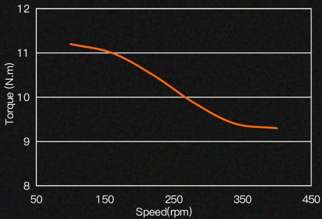
热平衡态T-N曲线 Thermal equilibrium state T-N curve ( 200mmX200mm铝散热板 )
