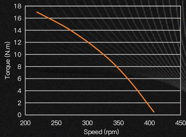
48V T-N曲线 (T-N under 48V)
