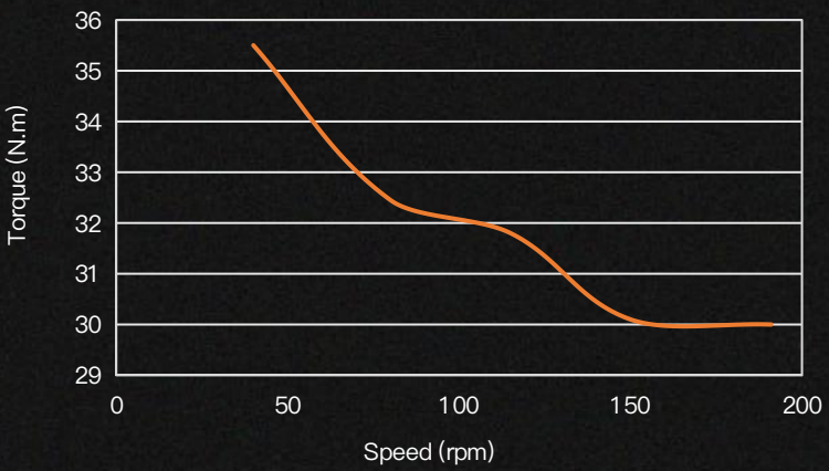
热平衡态T-N曲线 Thermal equilibrium state T-N curve ( 220mmx200mm铝散热板 )
