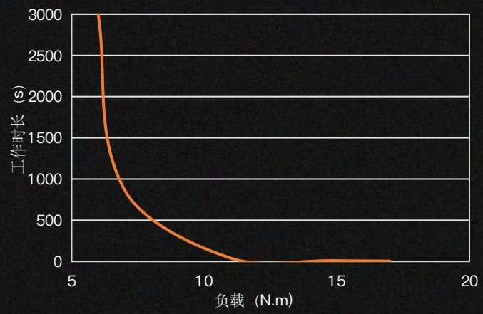
堵转工况最大过载曲线 ( Max Overload )
