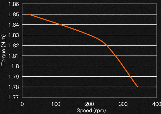
热平衡态T-N曲线 Thermal equilibrium state T-N curve ( 150mm×150mm铝散热板 )
