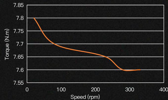
热平衡态T-N曲线 Thermal equilibrium state T-N curve ( 150mm×150mm铝散热板 )
