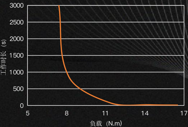
旋转工况最大过载曲线 ( Max Overload ) ( 150mm×150mm铝散热板 )
