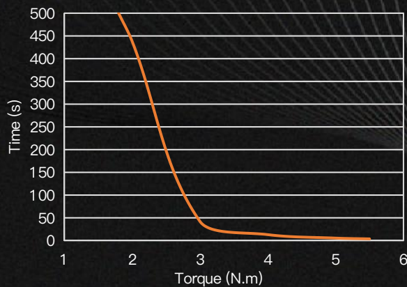
堵转工况最大过载曲线 ( Max Overload )
