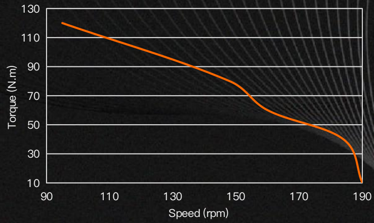
热平衡态T-N曲线 Thermal equilibrium state T-N curve ( 220mmx200mm铝散热板 )
