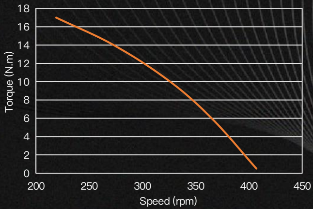
热平衡态T-N曲线 Thermal equilibrium state T-N curve ( 150mm×150mm铝散热板 )
