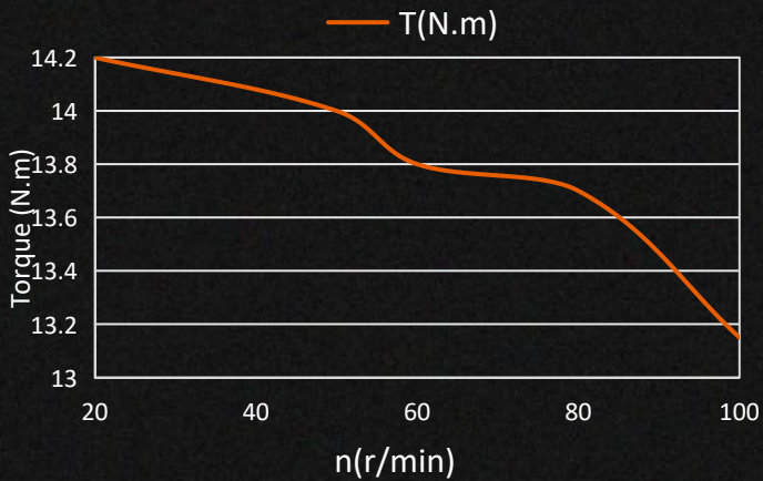
热平衡态T-N曲线 Thermal equilibrium state T-N curve ( 210mmX210mm铝散热板 )
