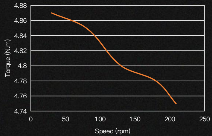
热平衡态T-N曲线 Thermal equilibrium state T-N curve ( 150mm×150mm铝散热板 )
