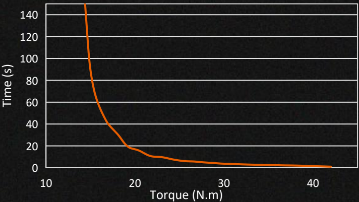
堵转工况最大过载曲线 ( Max Overload )
