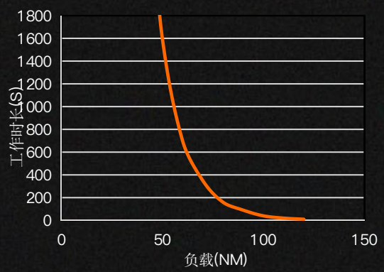
堵转工况最大过载曲线 ( Max Overload )
