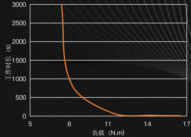
旋转工况最大过载曲线 ( Max Overload ) ( 150mm×150mm铝散热板 )
