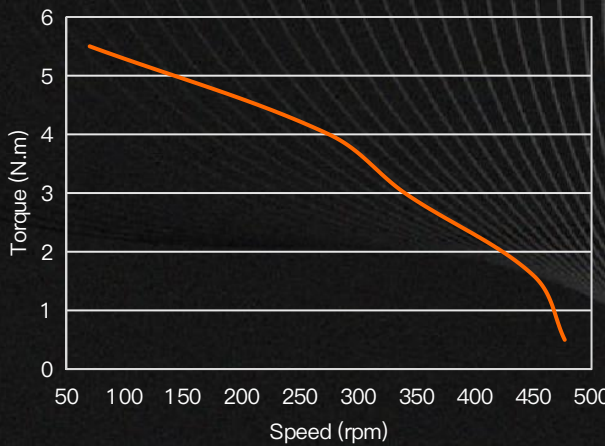
热平衡态T-N曲线 Thermal equilibrium state T-N curve ( 150mm×150mm铝散热板 )
