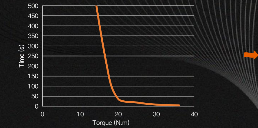
堵转工况最大过载曲线 ( Max Overload )
