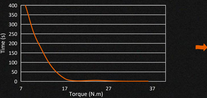
堵转工况最大过载曲线 ( Max Overload )
