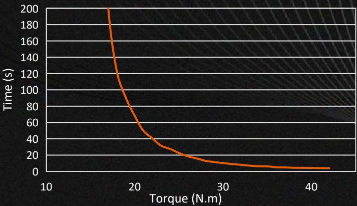
旋转工况最大过载曲线 ( Max Overload ) ( 210mm×210mm铝散热板 )
